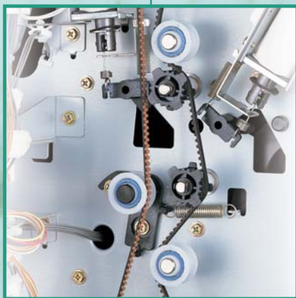
ベルトテンションプーリー
